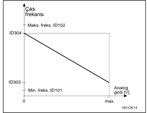
Şekil 8-11. Referans deęiřtirildi
