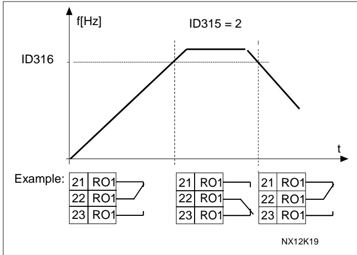
Şekil 8-16. Çıktı frekansı izleme
