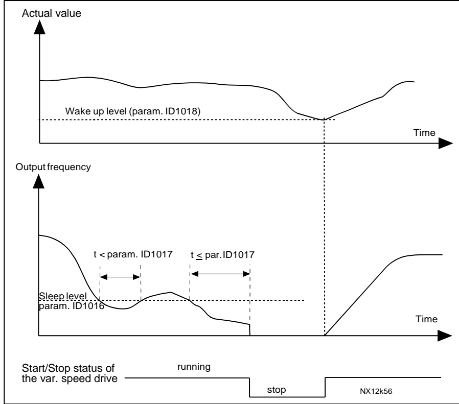
Şekil 8-56. Frekans dönüştürücü uyku işlevi
