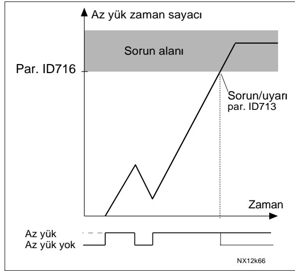
Şekil 8-52. Az yük zaman sayaç işlevi
