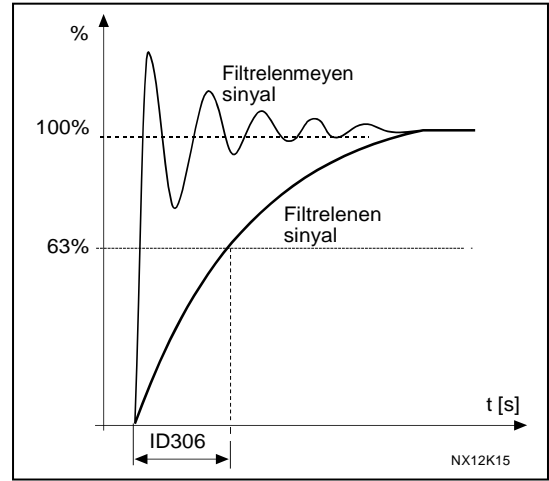
Şekil 8-12. Referans filtreleme
