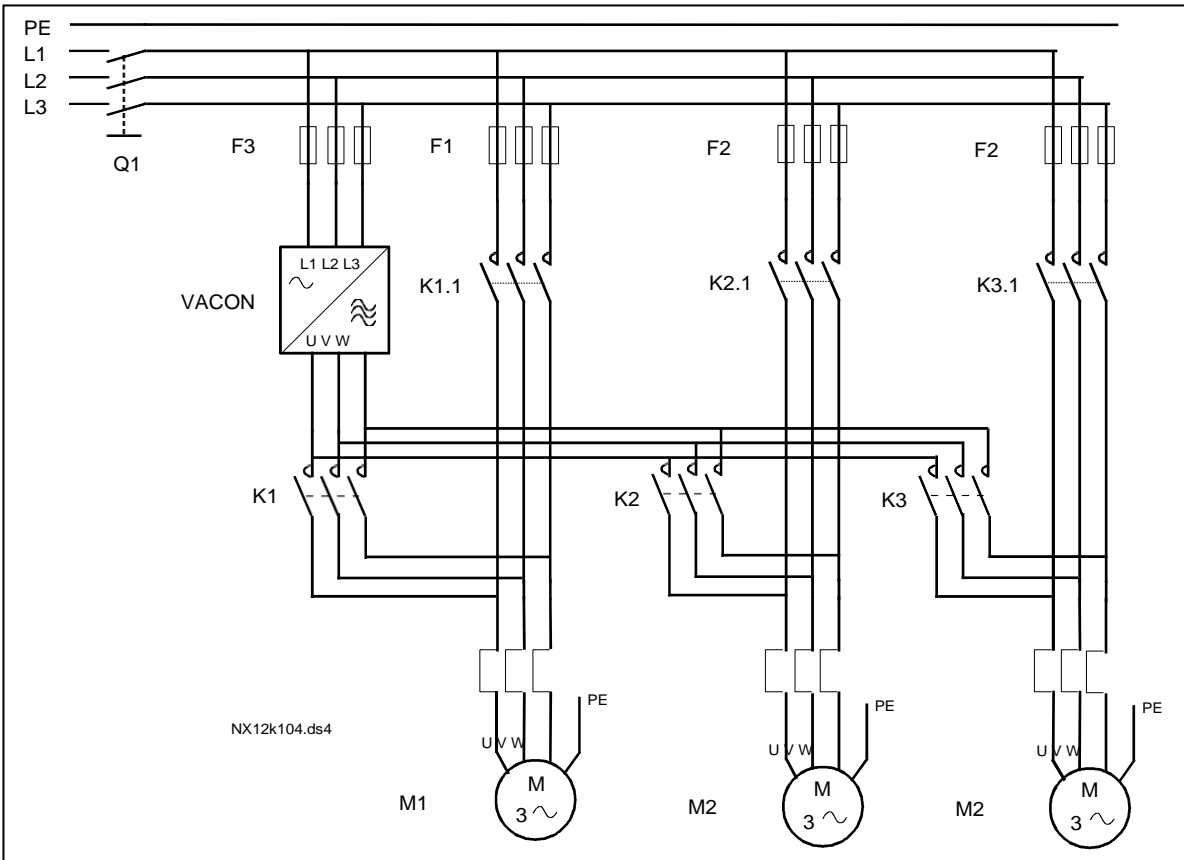
Şekil 7-6. 3-pompa otodeğiştir örneđi, ana şema
