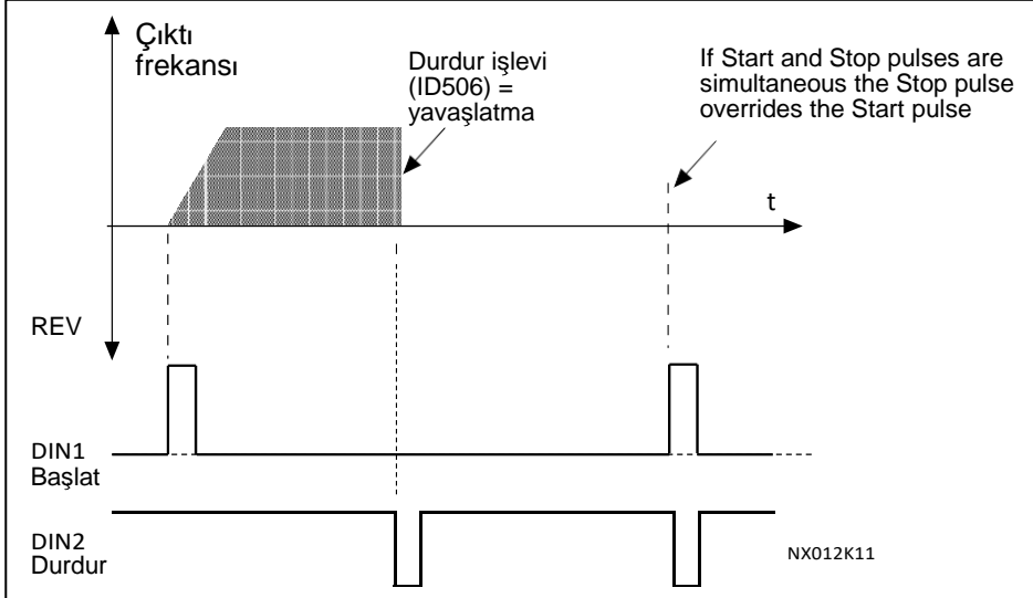
Şekil 8-8. Başlat vuruşu/Durdur vuruşu.
