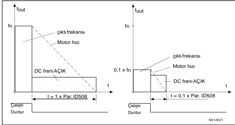
Şekil 8-43. Durdur modundayken DC-frenleme zamanı = Yavaslatma.
