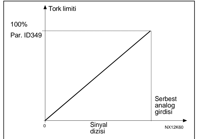
Şekil 8-39. Tork izleme limitinin azaltılması
