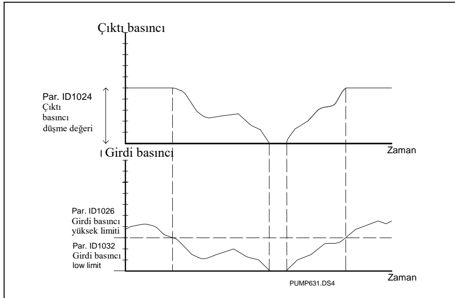
Şekil 8-60. Girdi basıncına ve parametre ayarlarına bağlı olarak çıktı basınç davranışı
