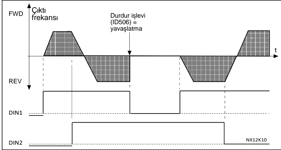
Şekil 8-7. Başlat, Durdur, Geri
