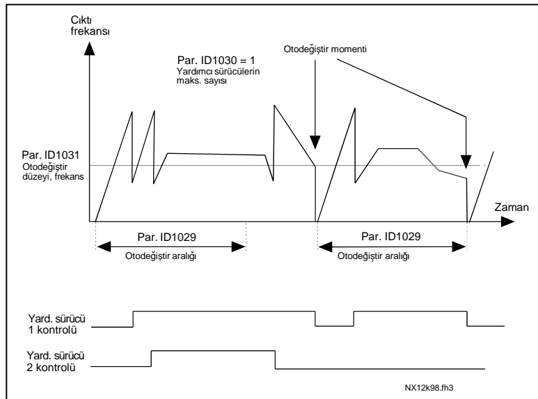
Şekil 8-64. Otodeğiştir aralık ve limitleri
