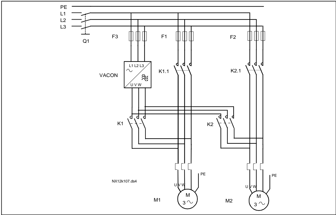
Şekil 7-5. 2-pompa otodeğiştir örneđi, ana şema
