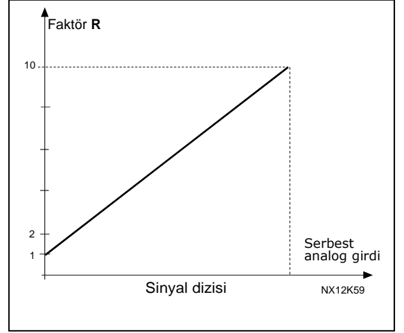
Şekil 8-28. Hızlanma ve yavaşlama zamanlarının azaltımı
