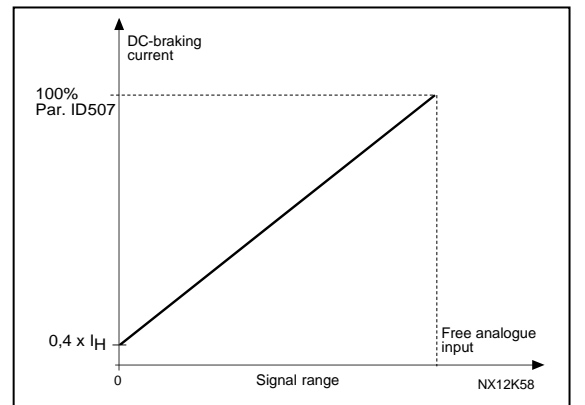
Şekil 8-27. DC frenleme akımının azaltılması
