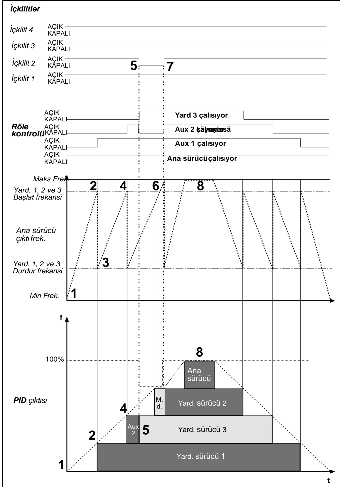
Şekil 7-4. Üç yardımcı sürücü ile PFC uygulamasının işlevinin örneği
