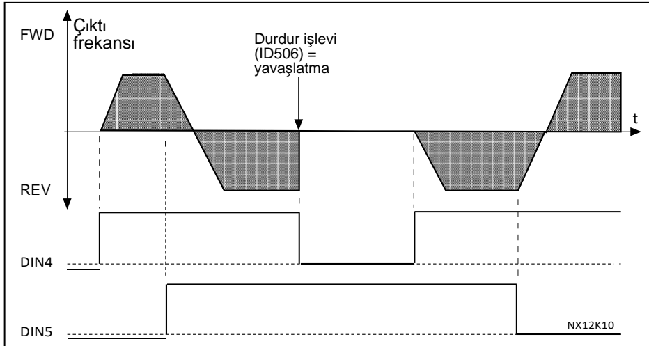
Şekil 8-31. Başlat,Durdur, Geri
