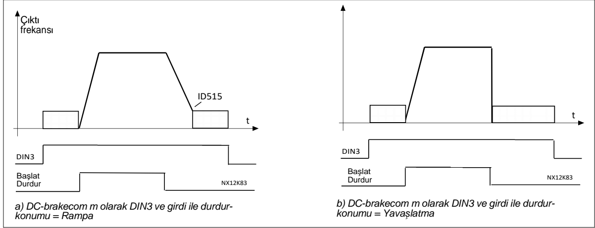
Şekil 8-9. DC-fren komutu girdisi olarak DIN3: a) Stop modu = Rampa, b) Stop modu = yavaşlatma
