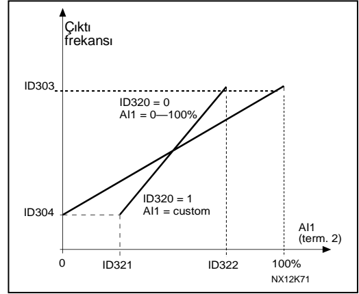
Şekil 8-18. AI1 sinyal deęiřtirme yok
