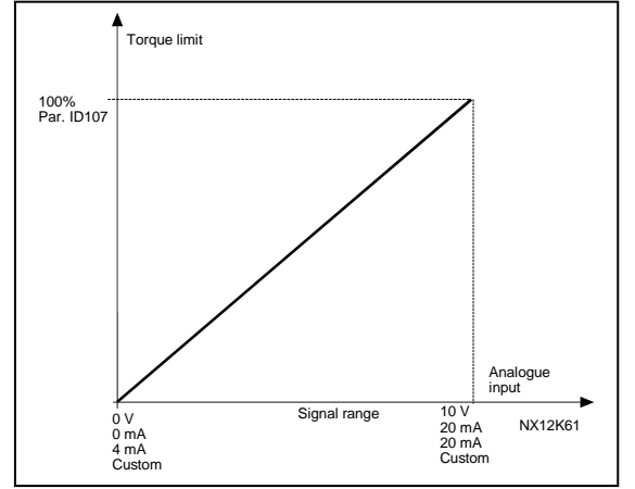
Şekil 8-26. Maks. motor akımının derecelendirmesi
