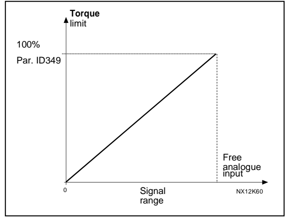
Şekil 8-29. Tork izleme limitinin azaltılması
