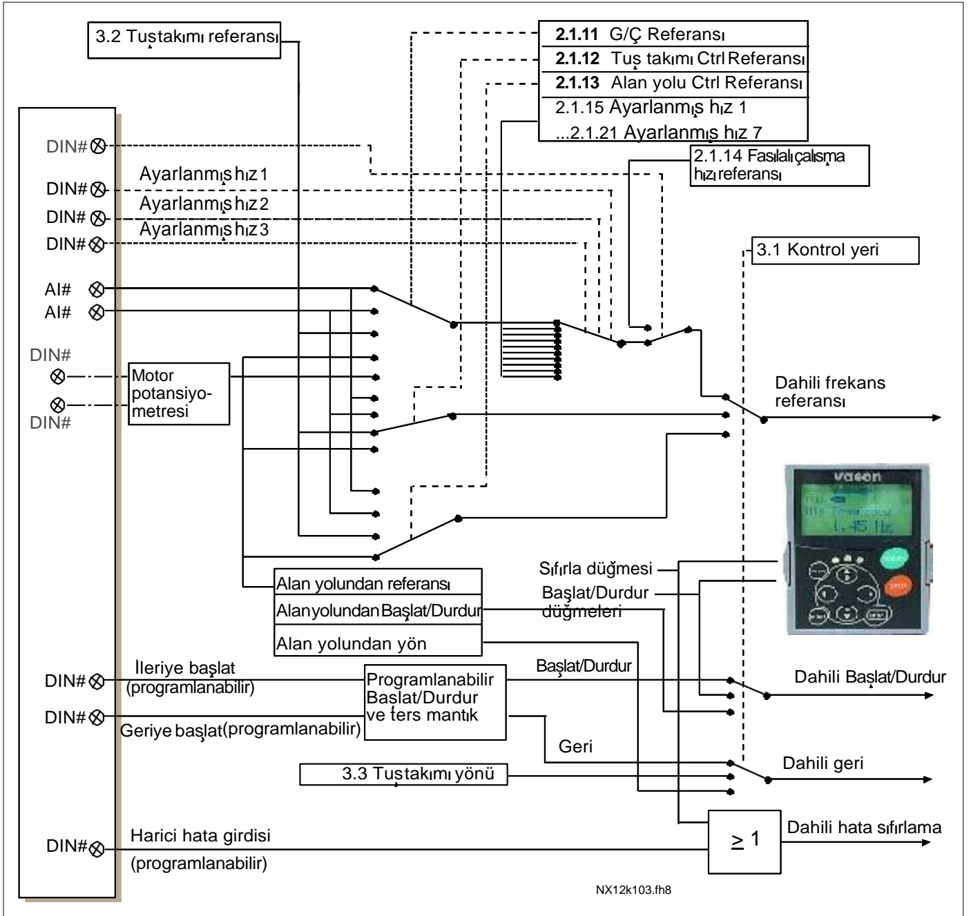
Şekil 6-1. Çok-amaçlı Kontrol Uygulamasının kontrol sinyal mantığı
