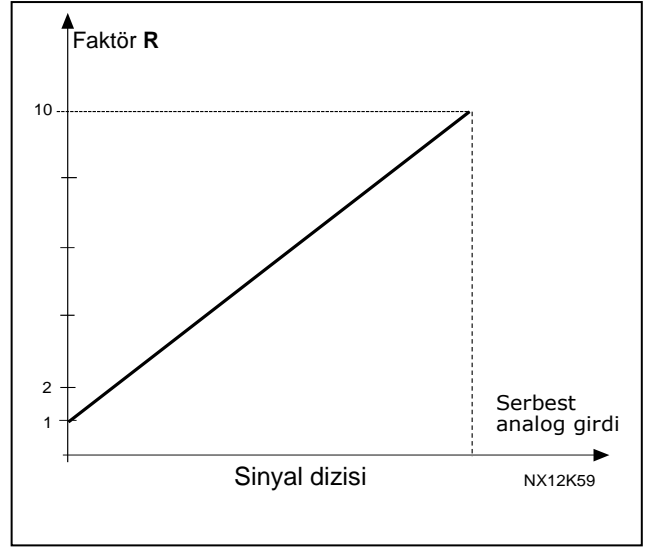
Şekil 8-38. Hızlanma ve yavaşlama zamanlarının azaltımı
