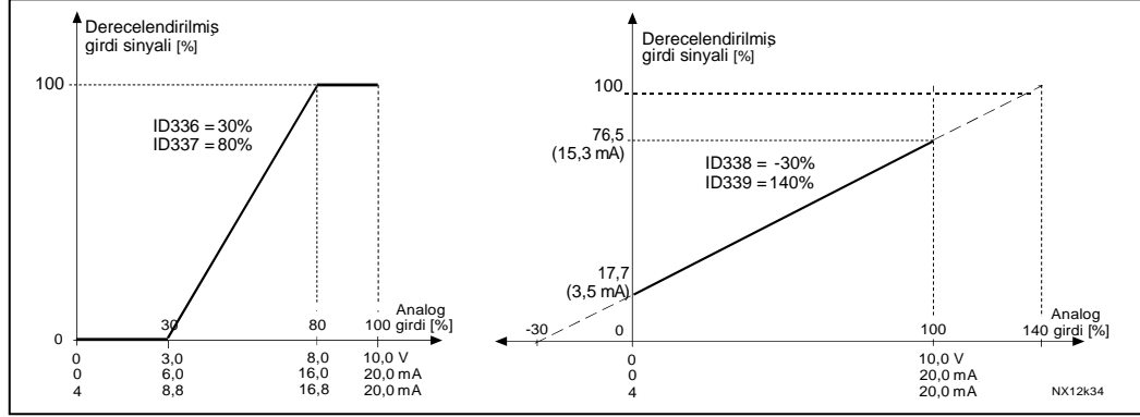
Şekil 8-22. Gerçek değer sinyal derecelendirme örnekleri
