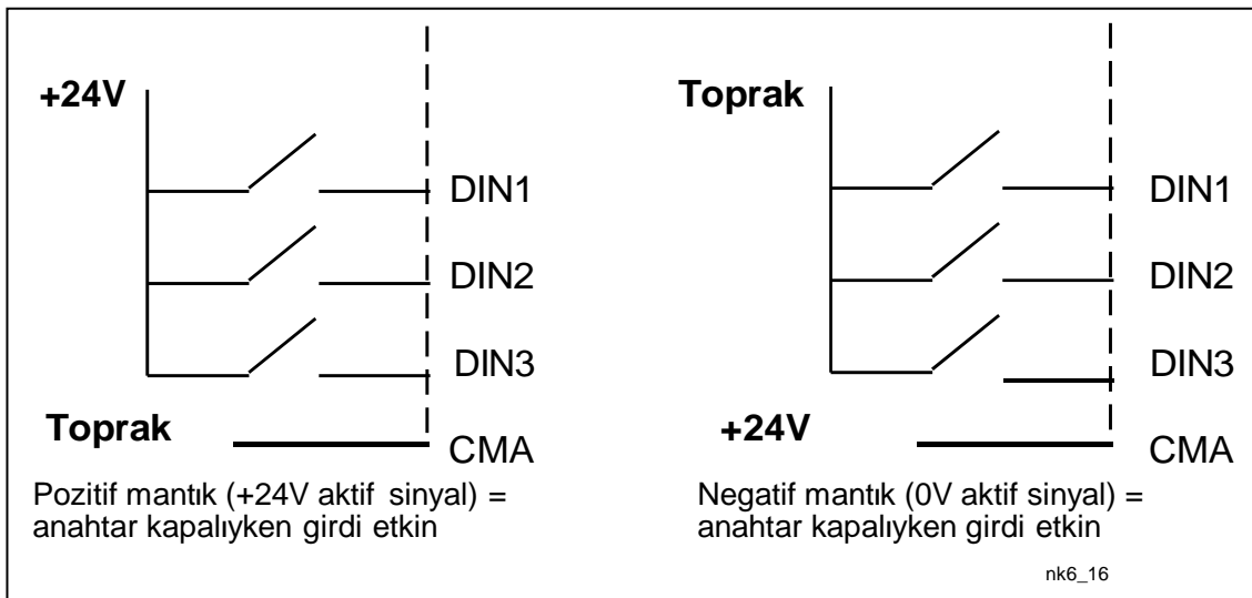
Şekil 6-26. Pozitif/Negatif mantık
