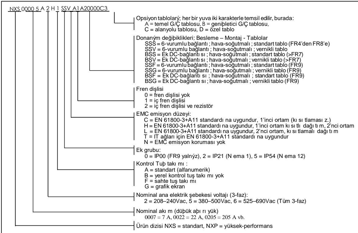
Şekil 3-1. Vacon NX tip adı kodu, FR4'den FR9'a çerçeveler
