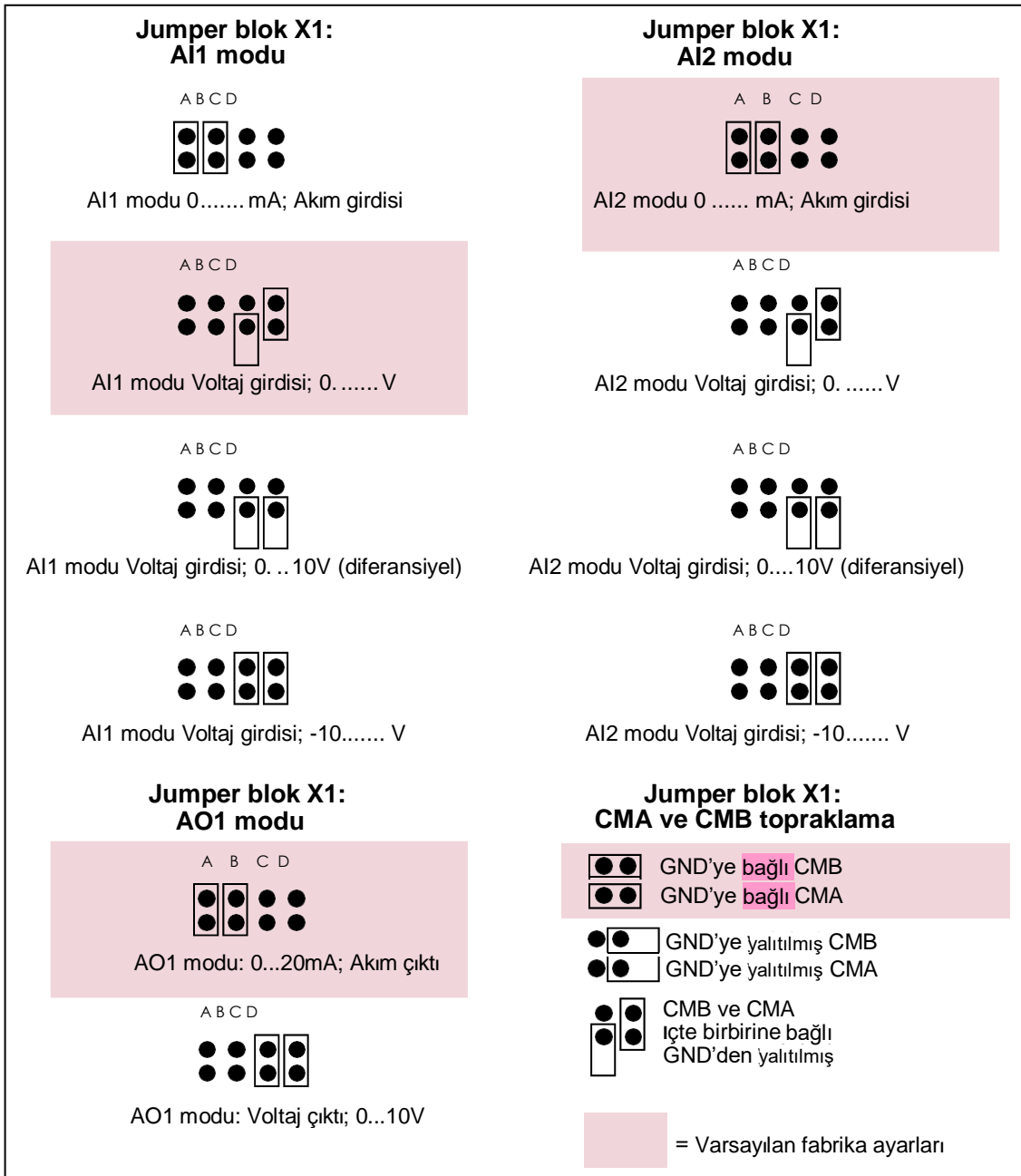
Şekil 6-28. NXOPTA1 için jumper seçimi
