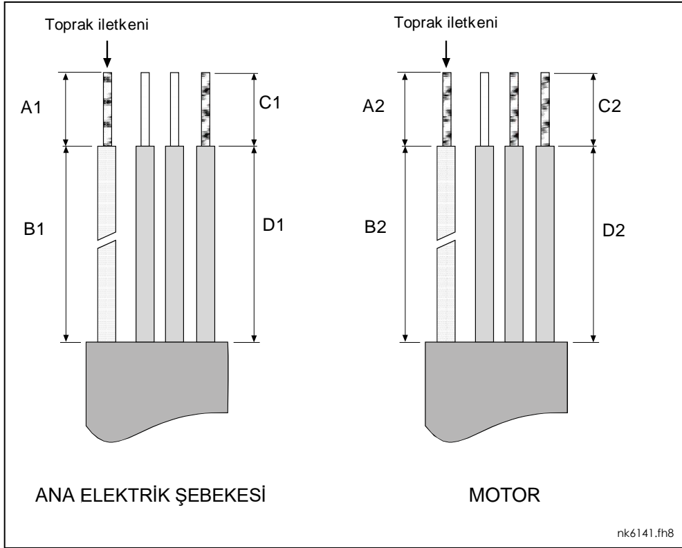
Şekil 6-4. Kabloların soyulması
