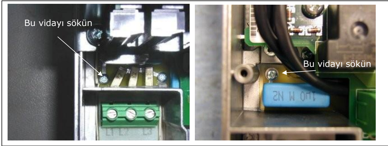
řekil 5-18. EMC koruma sınıfının deęiřtirilmesi, FR4 (sol) ve FR5 (saę).
