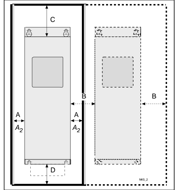
Şekil 5-10. Kurulum alanı
