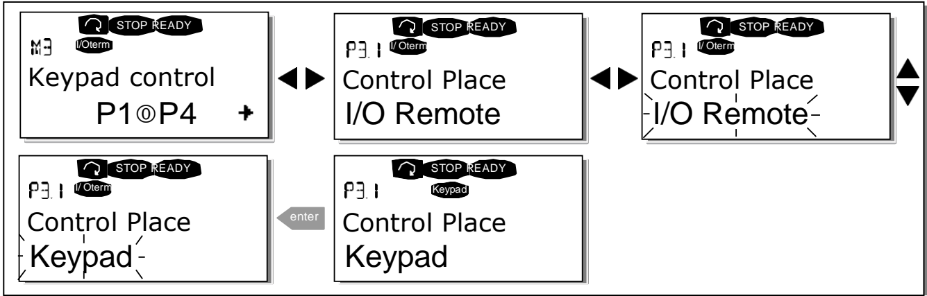
Şekil 7-6. Kontrol yerinin seçimi
