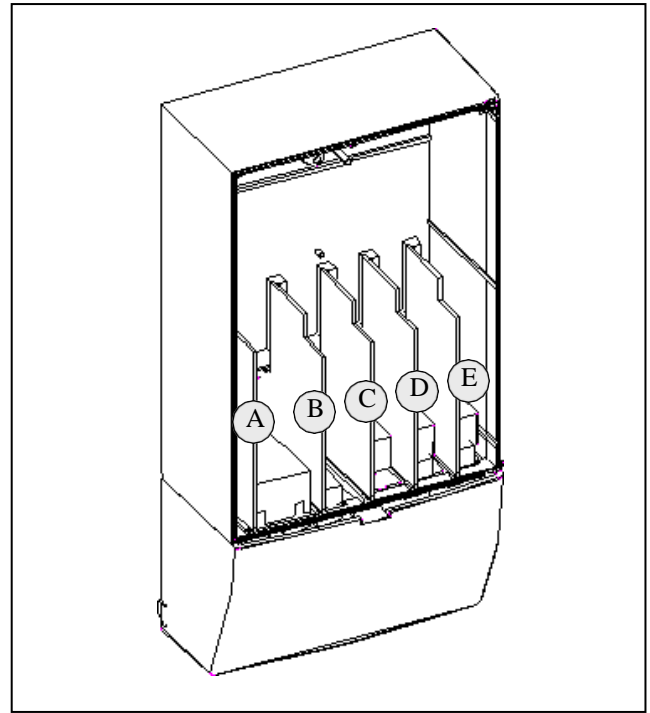
Şekil 6-20. Kontrol tablosu üzerinde temel ve opsiyon tablo bağlantıları
