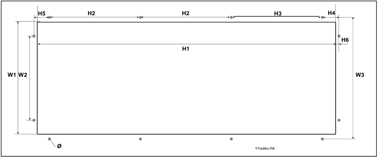
Şekil 5-5. Flanş kurulumu için gerekli açıklık, FR7/ FR8
